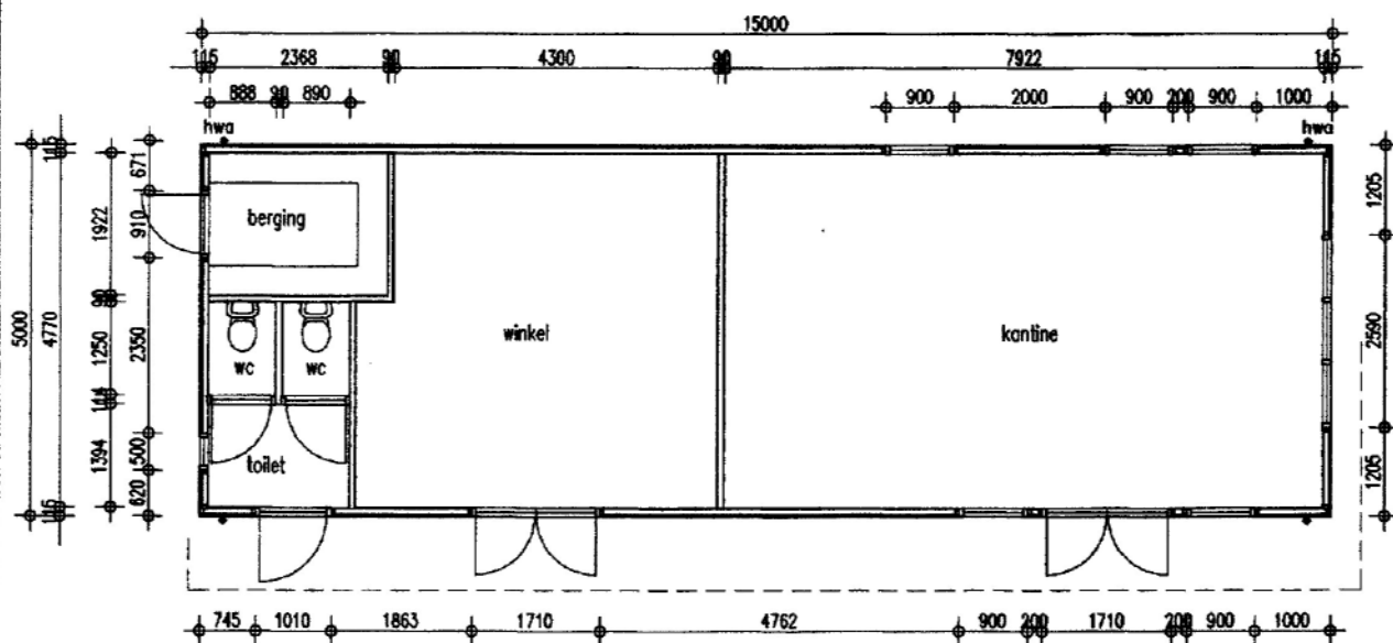
Plattegrond
