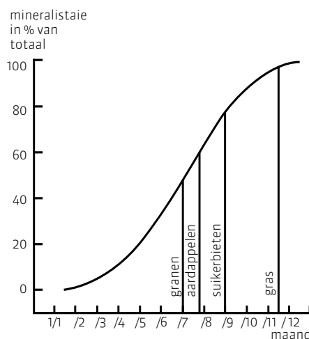
Figuur 2. De stikstof die gedurende het jaar vrijkomt en de mogelijke benutting door verschillende gewassen.
