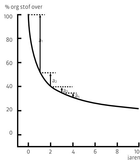
Figuur 1. De afbraak van organische stof uit stalmest onder veldproefomstandigheden.
